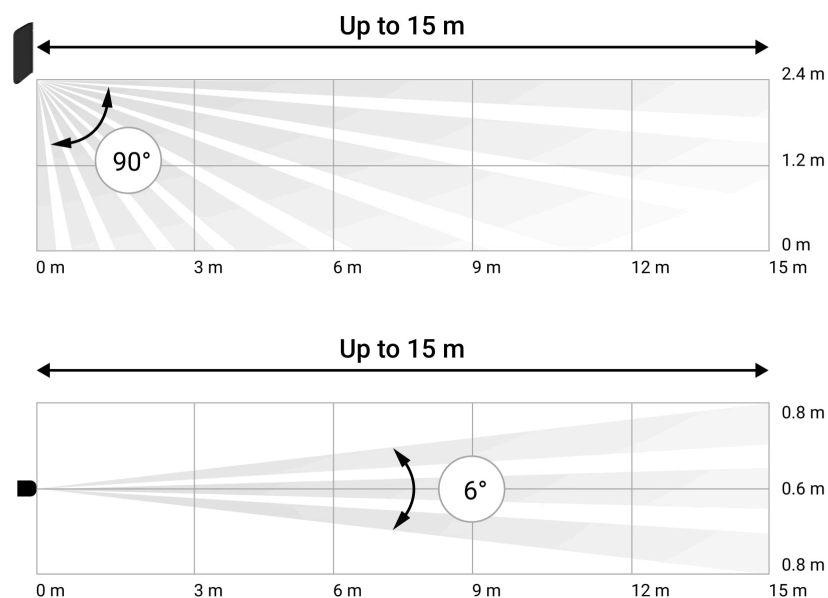
Angoli di rilevamento orizzontali e verticali
